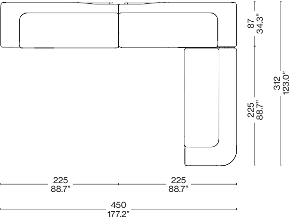
580 AB 01 + 580 AB 02+ 580 B2 02
