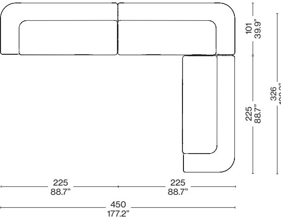
580 B2 01 + 580 B2 02+ 580 B2 02
